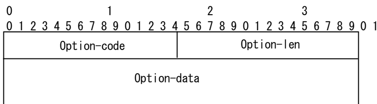
図 4-4 DHCPv6オプションフォーマット
