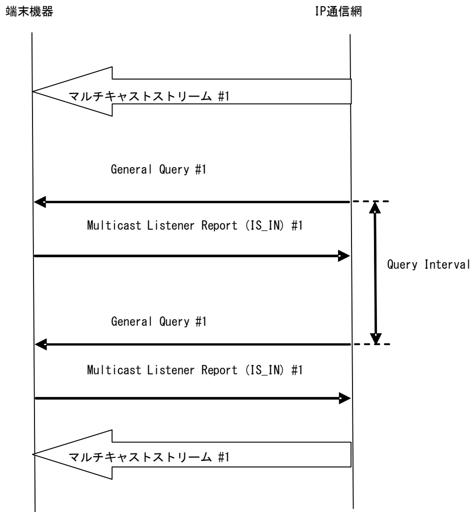
図 4-9 マルチキャスト受信継続確認シーケンス例
