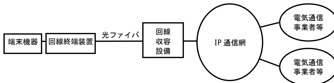
図 1-1 フレッツ 光25Gの基本構成
