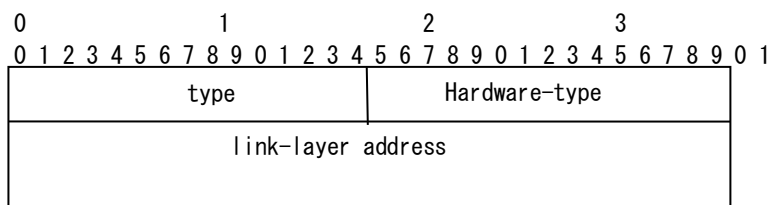
図 2-3 DUID-LLフォーマット
