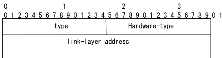
図 4-2 DUID-LLフォーマット
