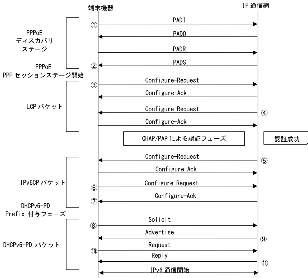
図 5-3 接続シーケンス (例)
