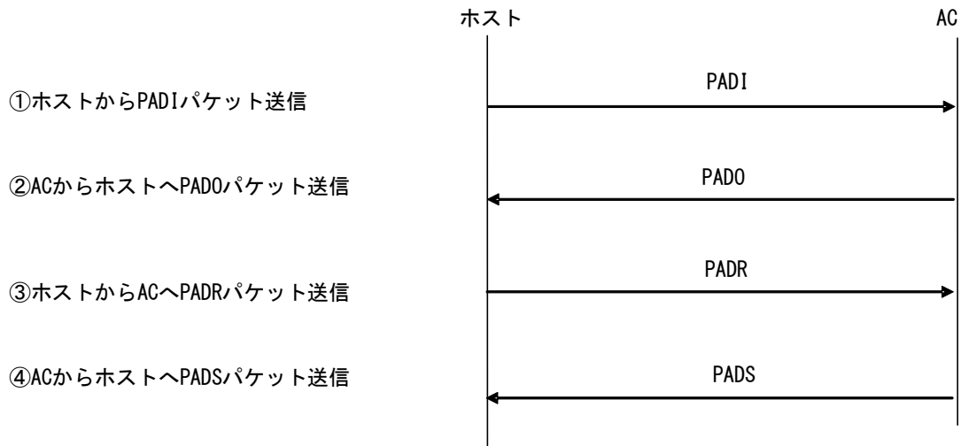
図 5-1 PPPoEセッション確立手順
