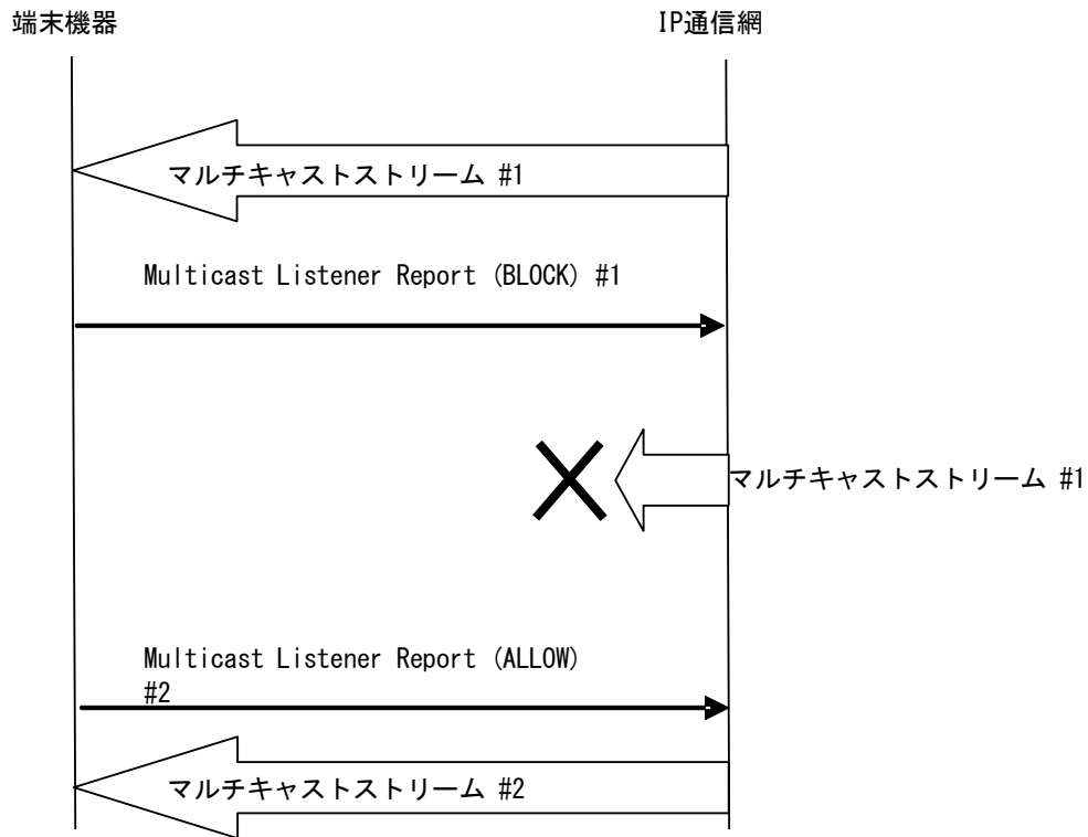
図 4-10 チャンネル切り替えシーケンス例
