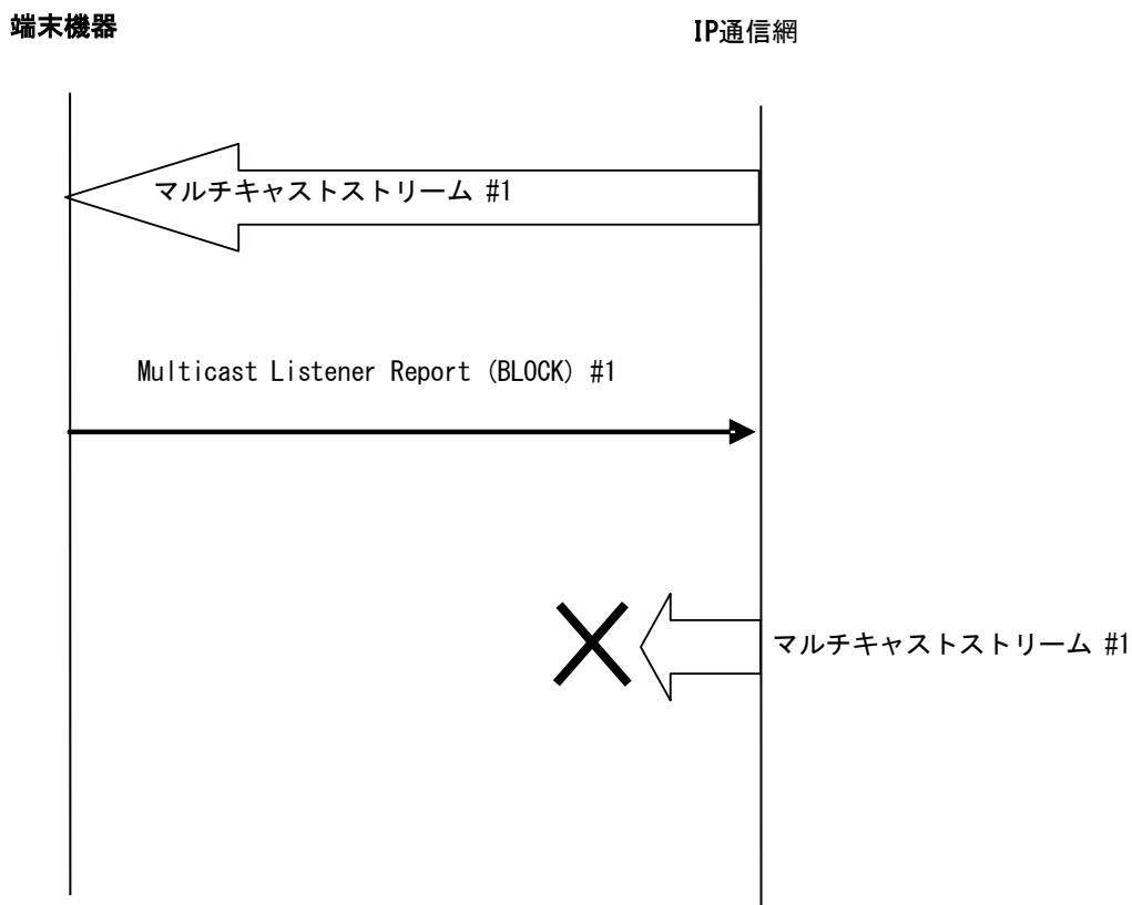
図 2-11 マルチキャスト受信停止シーケンス例
