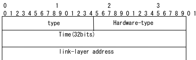
図 4-3 DUID LLTフォーマット
