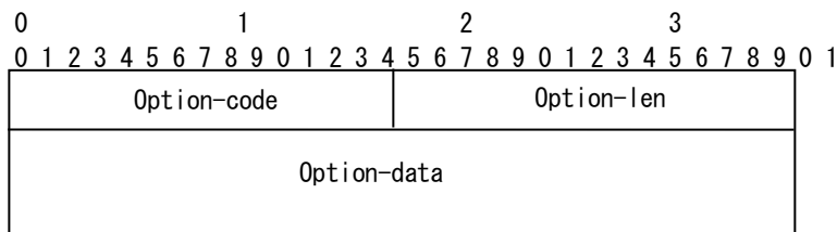
図 2-3 DHCPv6オプションフォーマット
