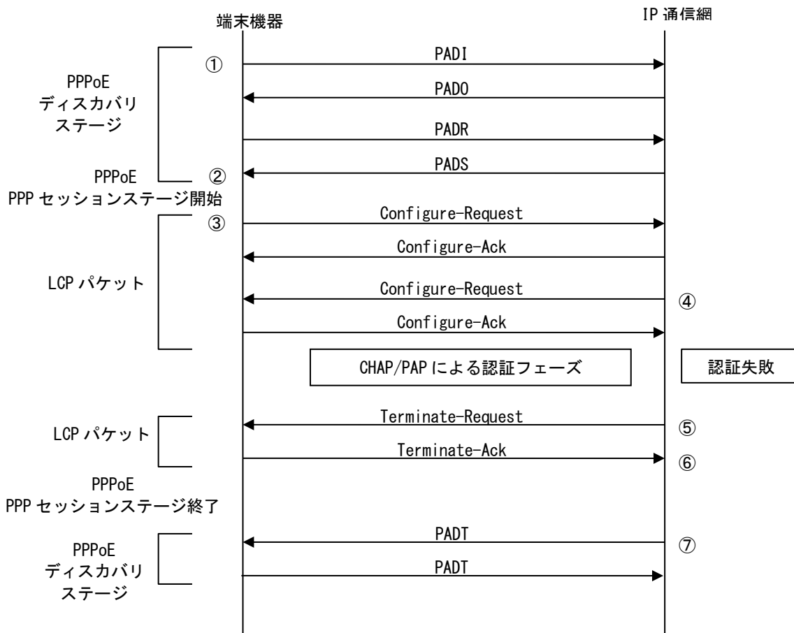
図 5-5 認証失敗シーケンス (例)
