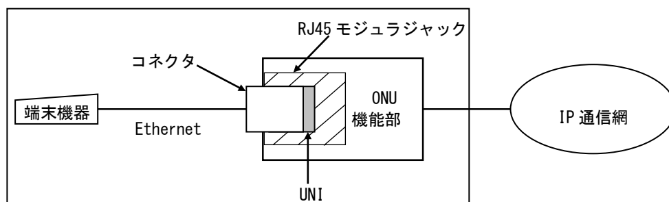
図 4-1 フレッツ 光ネクストのインターフェース規定点
