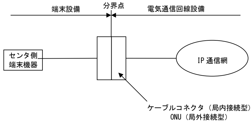
図1-5 フレッツ・キャストの分界点
