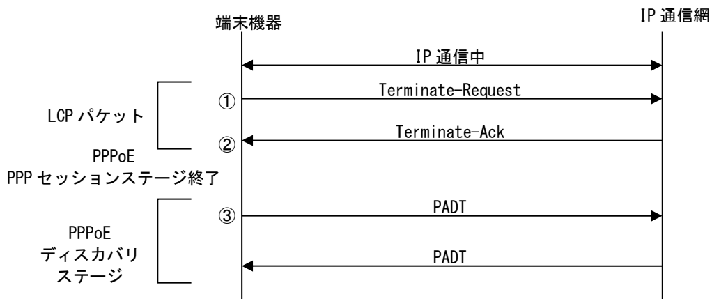
図 5-4 切断シーケンス (例)
