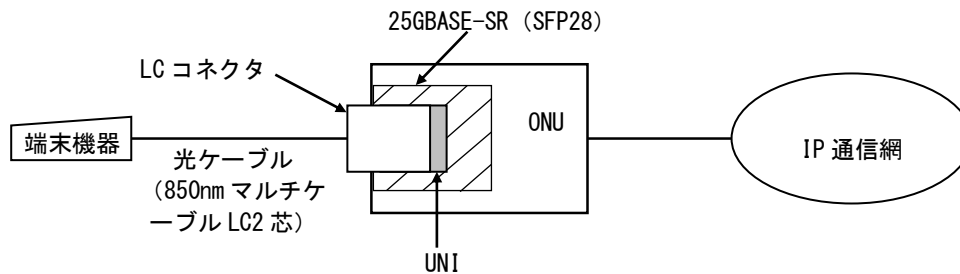
図 1-3 フレッツ 光25Gのインタフェース規定点
