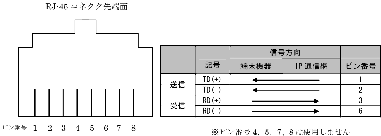
図 2-2 コネクタ先端面から見た RJ-45 コネクタのピン配置
