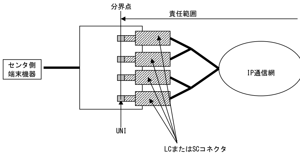
図 1-7 本サービスにおける施工・保守上の責任範囲分界点
