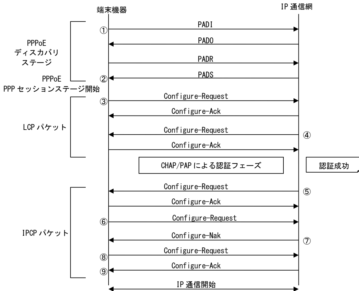
図 5-2 接続シーケンス (例)
