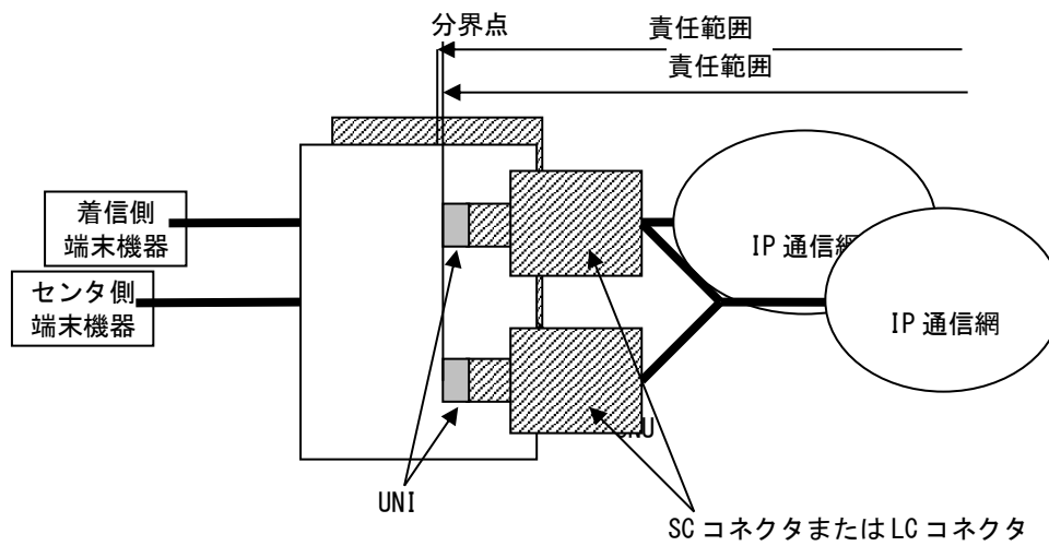
図 1-8 フレッツ・キャスト（局内接続型）における施工・保守上の責任範囲分界点
