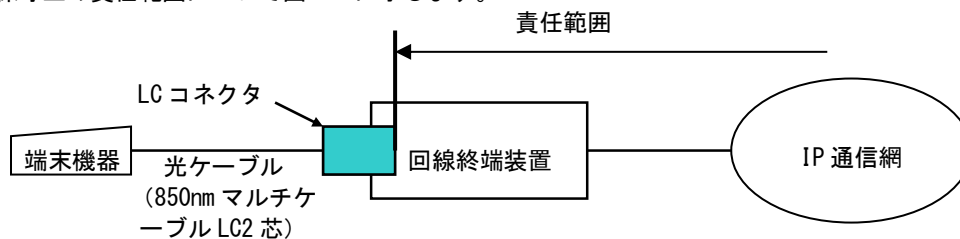
図 1-5 施工・保守上の責任範囲
