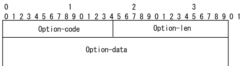
図 2-4 DHCPv6オプションフォーマット
