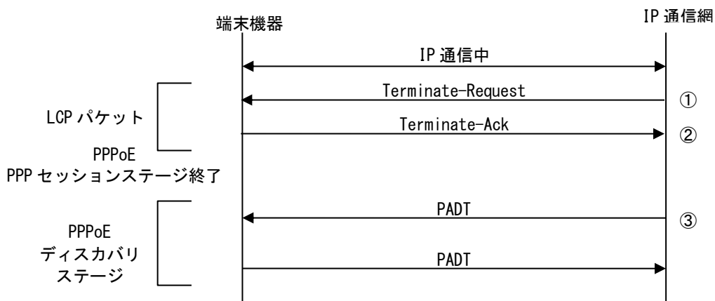
図 5-6 強制切断シーケンス (例)
