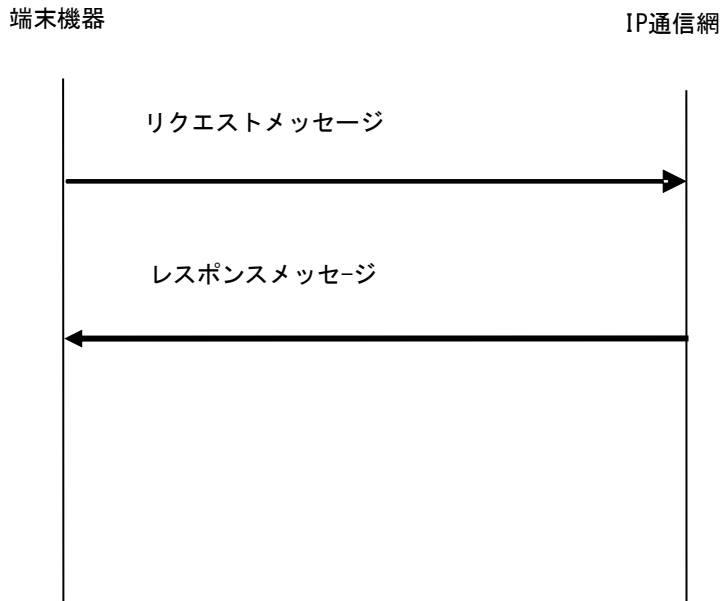
図 4-15 経路情報提供サーバとの通信シーケンス
