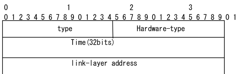
図 2-2 DUID LLTフォーマット
