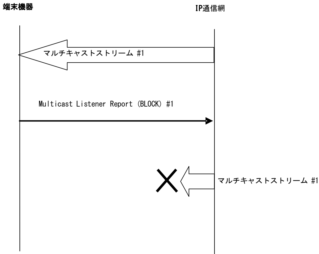
図 4-11 マルチキャスト受信停止シーケンス例
