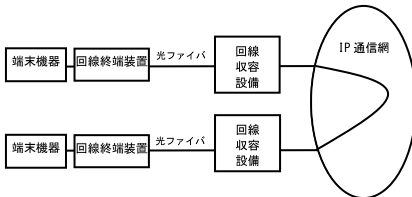
図 3-2 フレッツ・v6オプションの契約者同士の通信
